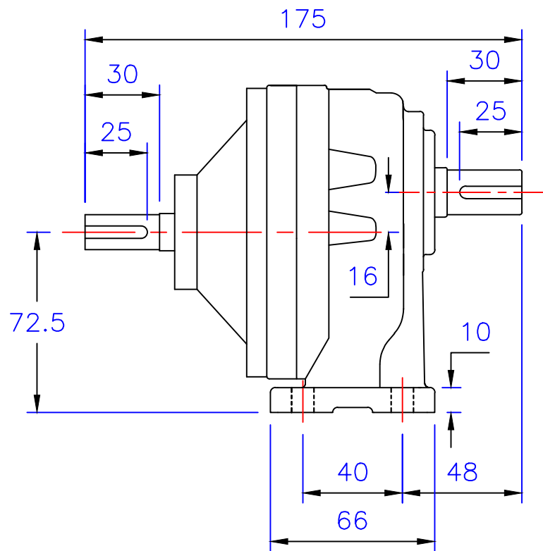
入力轴 Input shaft
